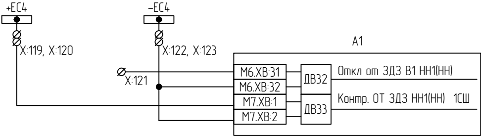
Цепи ввода (НН, СН) А1
