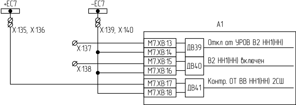
Цепи ввода (НН, СН) А1
